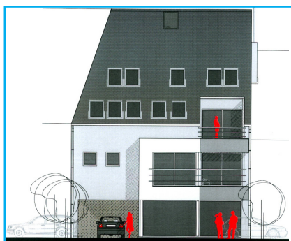
tekening vooraanzicht
